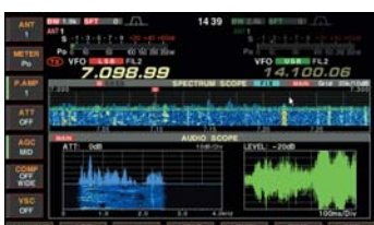
Mini spectrum scope and audio scope
